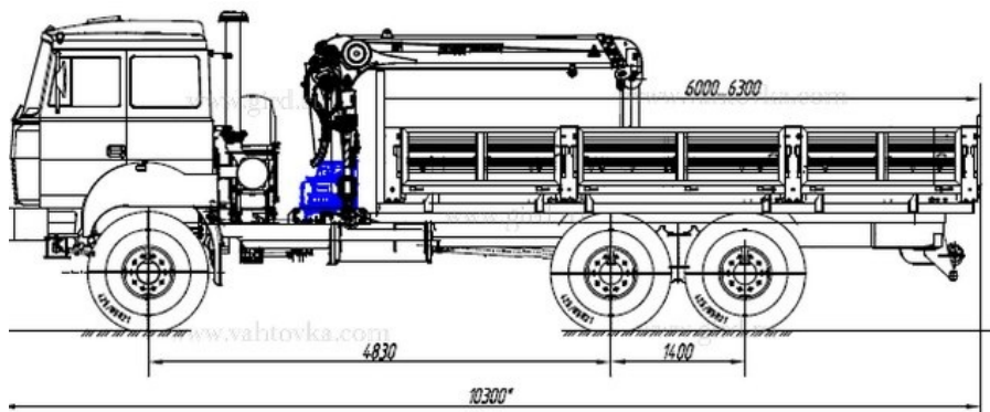
Технические характеристики шасси
