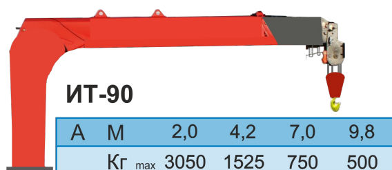
Крано-манипуляторная установка ИТ-90
