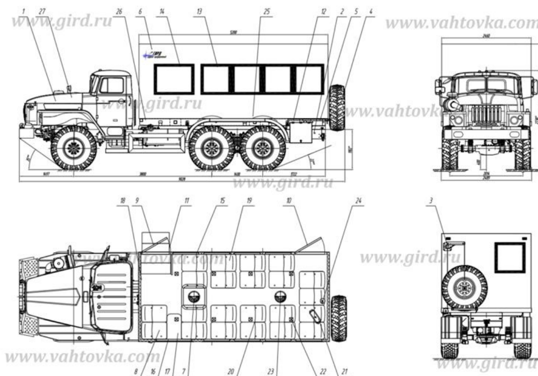
Схематический рисунок
