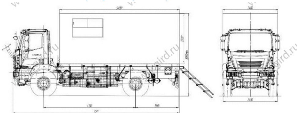
Схематический рисунок Транспортно бытового автомобиля
