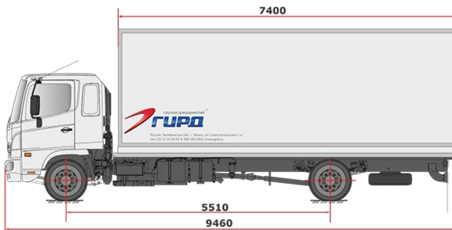
Схематический рисунок HINO 500 GH8JPTA-QHR
