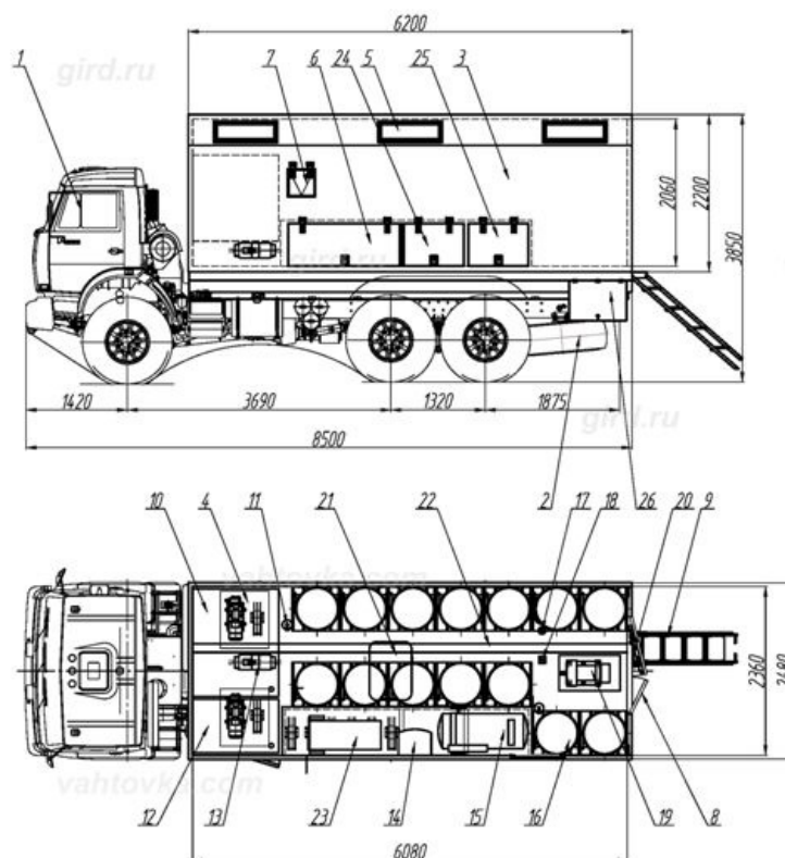
Схематический рисунок
