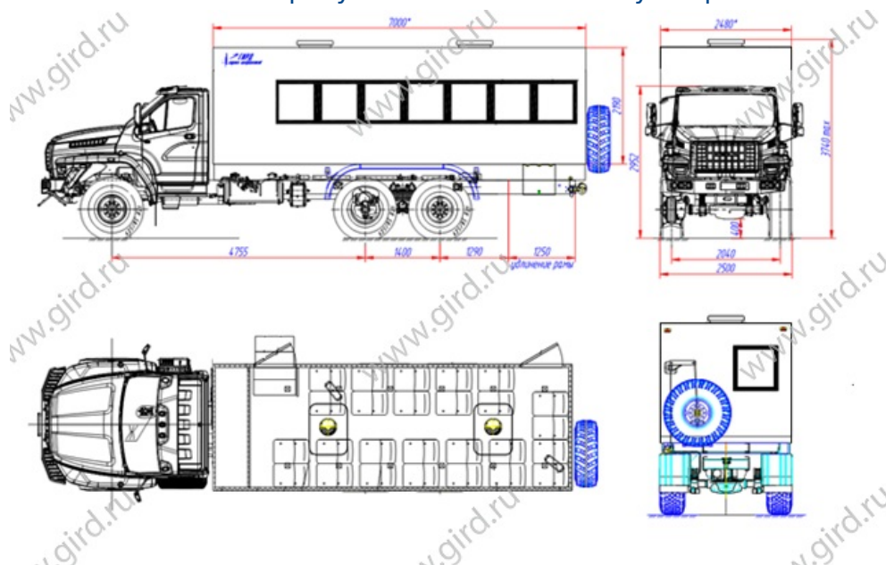
Схематический рисунок вахтового автобуса Урал NEXT
