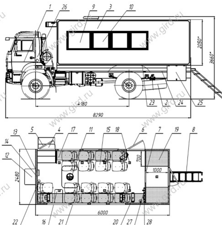
Схематический рисунок Вахтового автобуса
