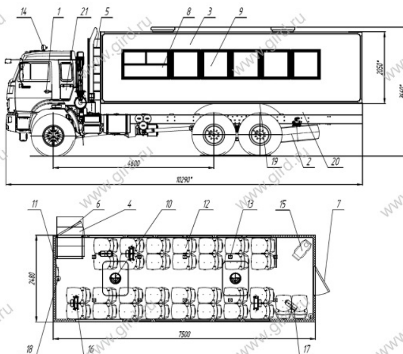
Схематический рисунок Вахтового автобуса
