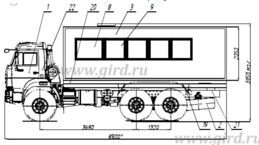
Схематический рисунок
