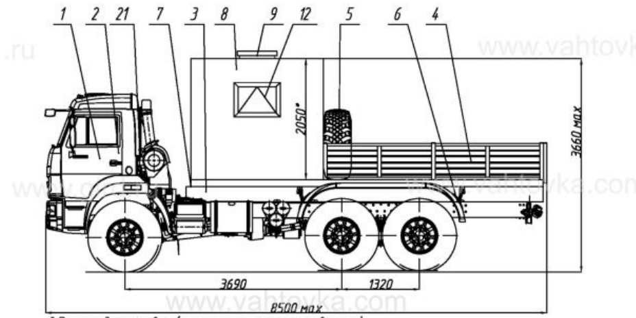
Схематический рисунок
