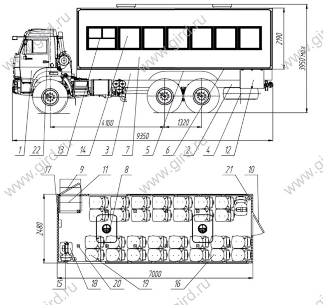
Схематический рисунок Вахтового автобуса
