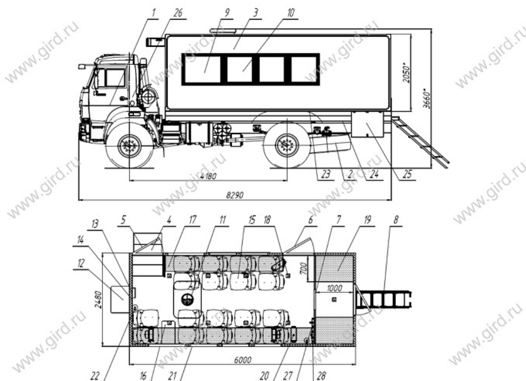
Схематический рисунок Вахтового автобуса
