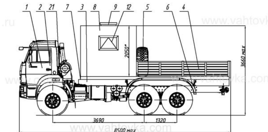
Схематический рисунок
