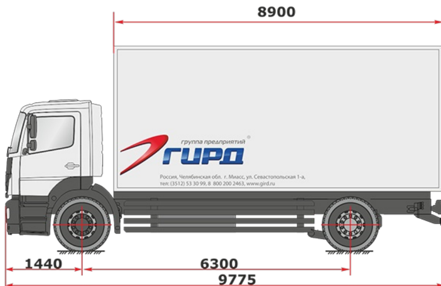
Схематический рисунок Mercedes-Benz Ахор 1824L
