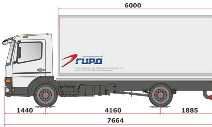
Схематический рисунок Mercedes-Benz Atego 1218L
