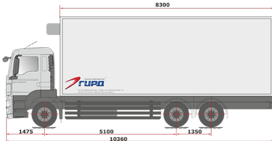
Схематический рисунок MAN TGS 26.400
