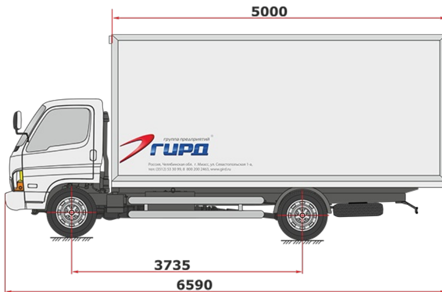
Схематический рисунок Hyundai HD-78 S.Cab
