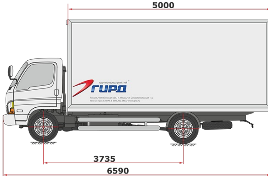
Схематический рисунок Hyundai HD-78 Long
