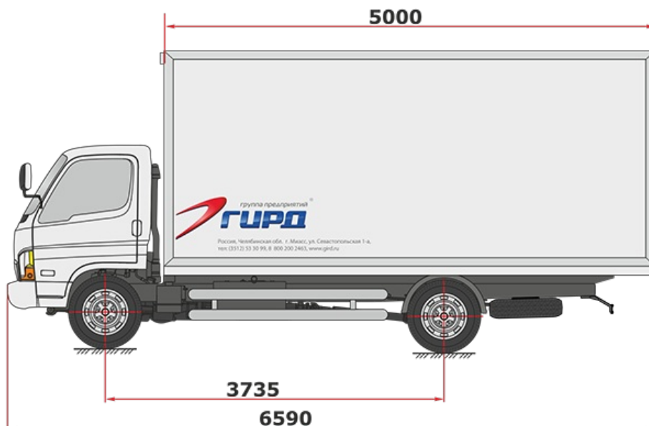
Схематический рисунок Hyundai HD-78 Long
