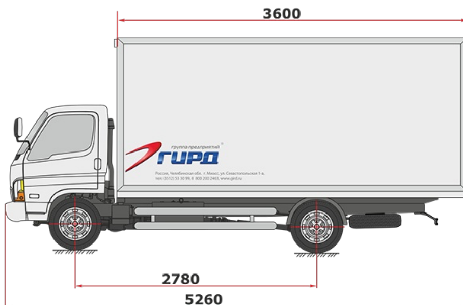
Схематический рисунок Hyundai HD-78 Short
