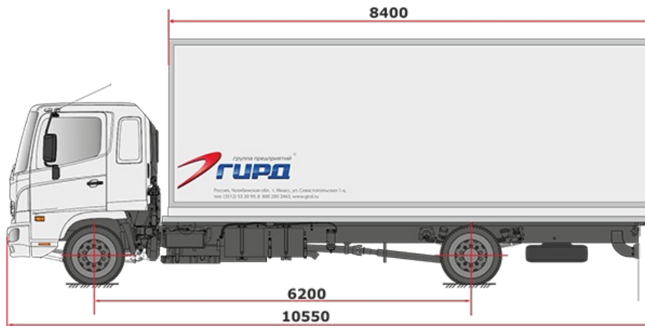
Схематический рисунок HINO 500 GH8JSTG-THR
