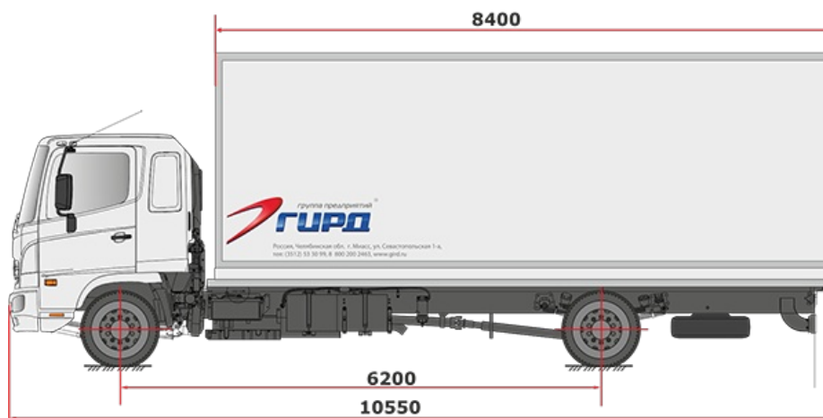
Схематический рисунок HINO 500 GH8JSTA-QHR
