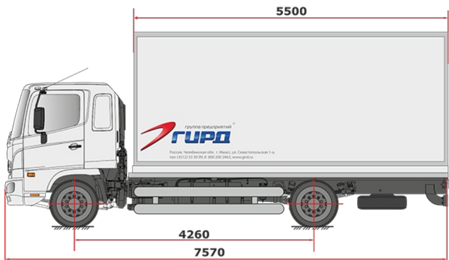
Схематический рисунок HINO 500 GH8JTG-QHR
