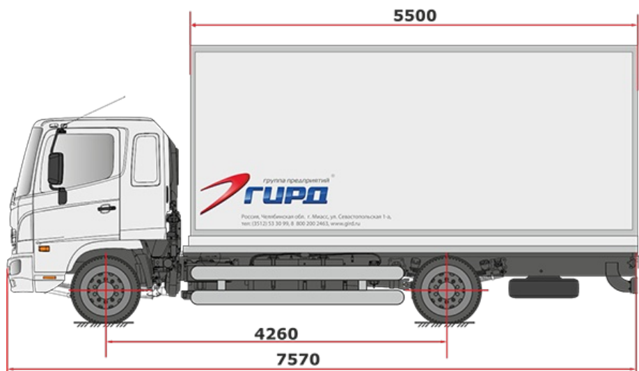
Схематический рисунок HIHO 500 GH8JJTA-QHR
