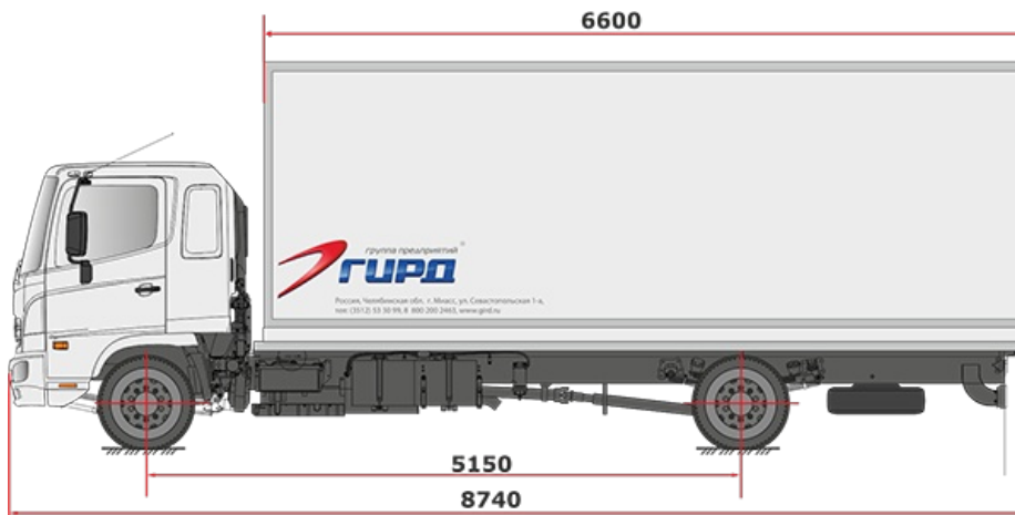
Схематический рисунок HINO 500 GD8JMTA-QHR
