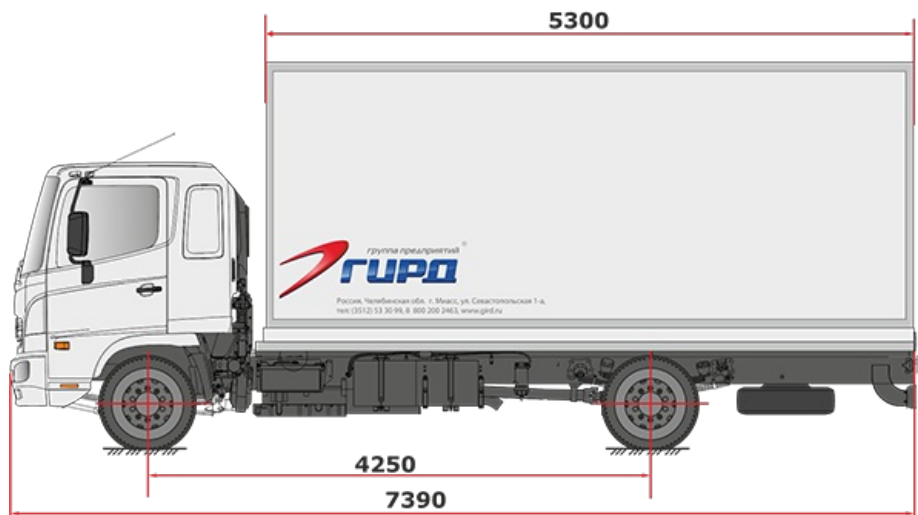
Схематический рисунок HINO 500 GD8JTG-QHR
