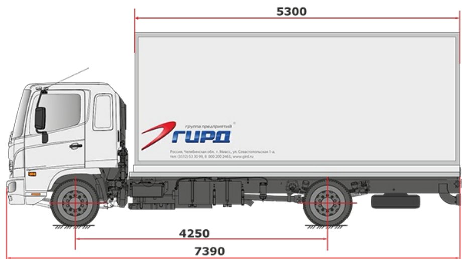
Схематический рисунок HIHO 500 GD8JTA-QHR
